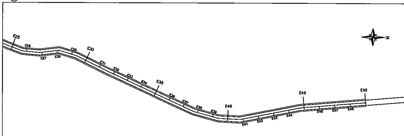
ESTAQUEAMENTO - ESTACA 25 A 49 SPT 139/4.4
